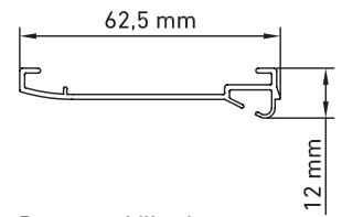
Barra estabilizadora Stabilising bar Barre stabilisatrice
